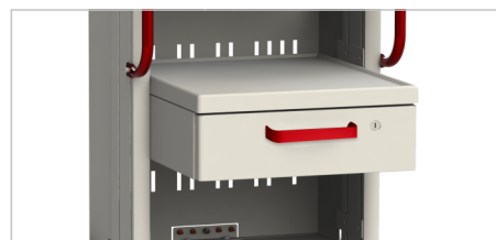
Ящик с замком (принадлежность) Внутренний размер (ш/г/в): 440x330x91 мм
