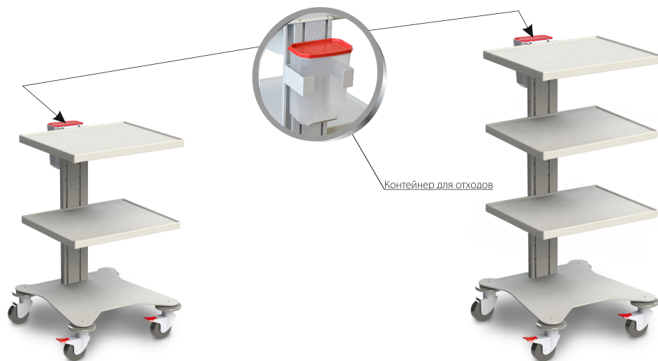
CA-6 509.305 Габариты (ш/г/в): 580x620x904 мм Размер полки (ш/г): 490x400 мм
